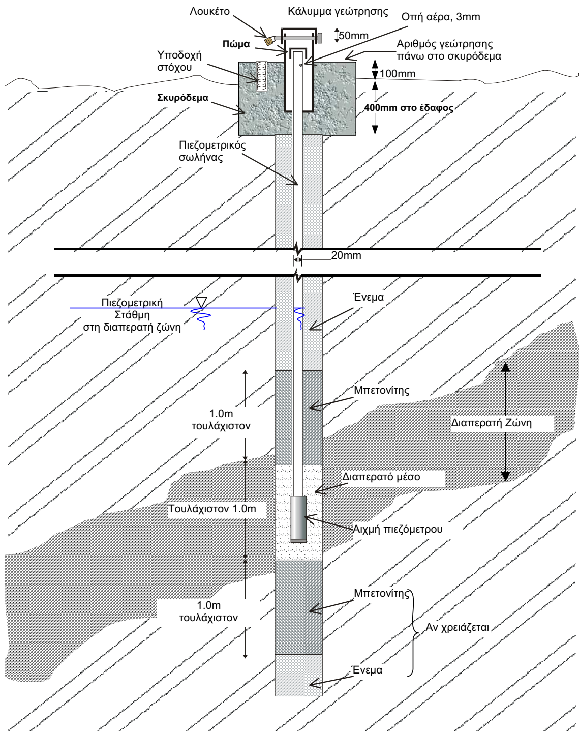
Σχήμα 2. Τυπική τομή πιεζόμετρου τύπου Casagrande
