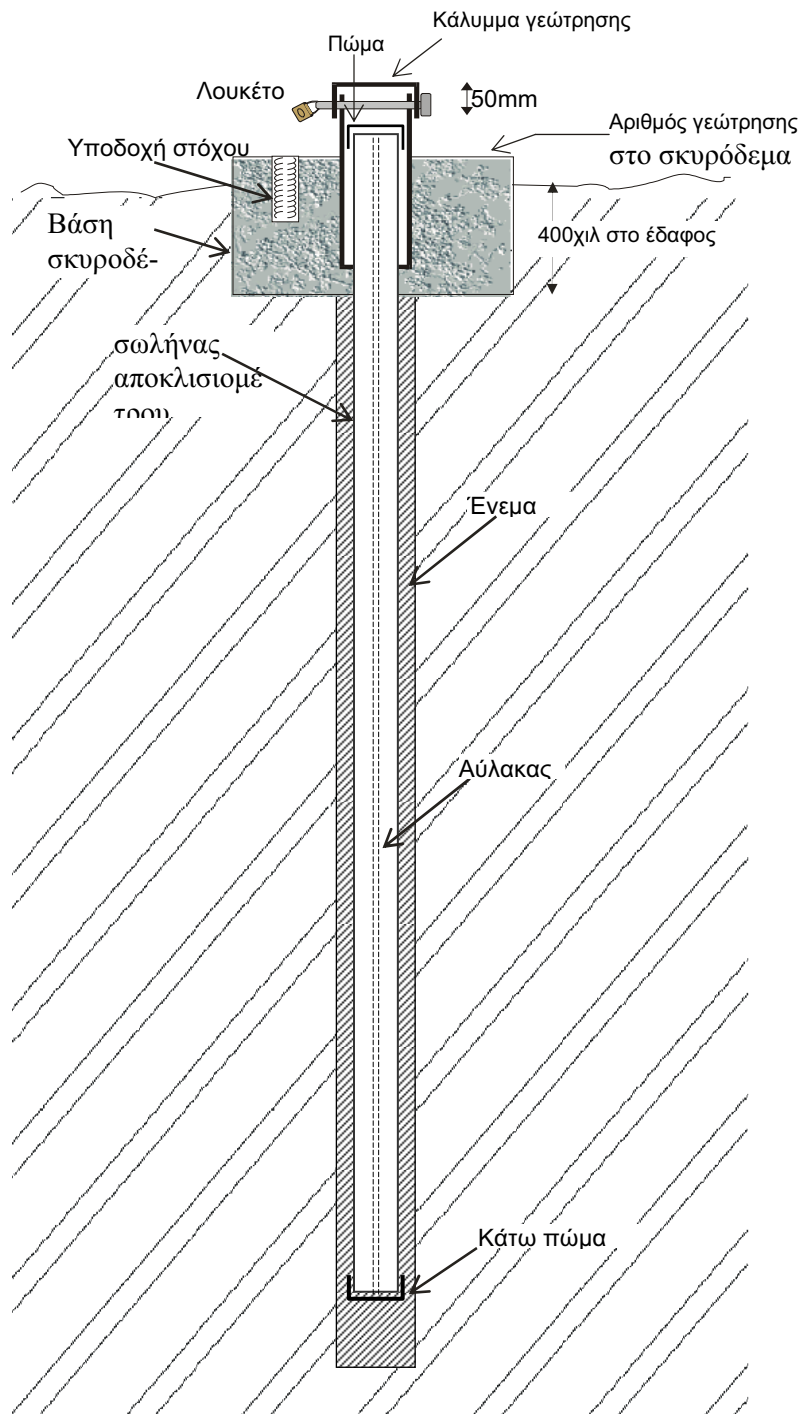
Σχήμα 3: Τυπική τομή αποκλισημέτρου
