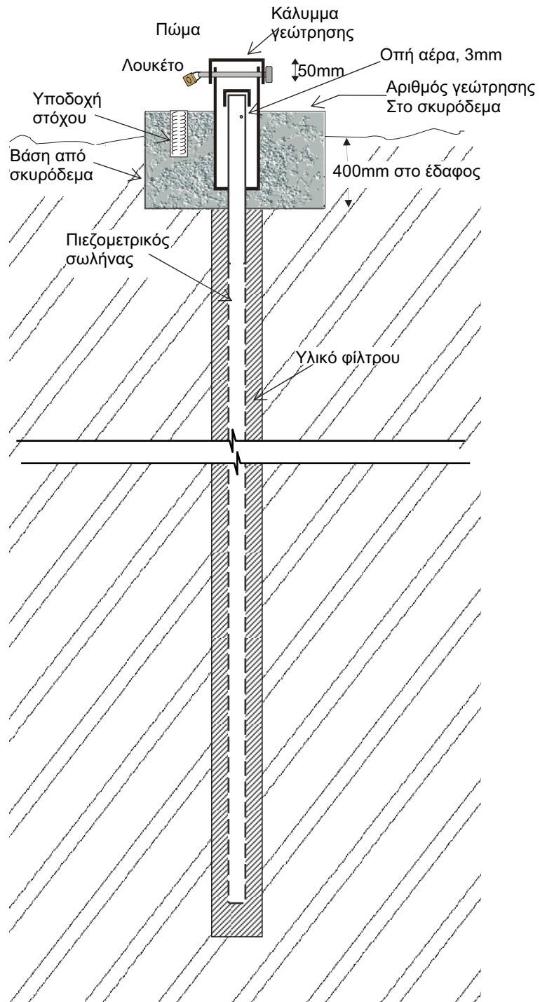
Σχήμα 1. Τυπική τομή πιεζομέτρου απλού τύπου
