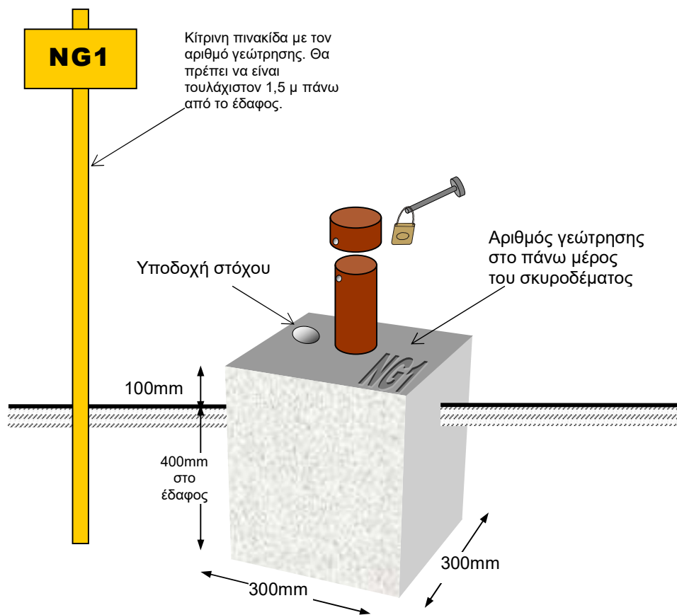
Σχήμα 4: Σκαρίφημα κεφαλής γεωτεχνικού οργάνου
