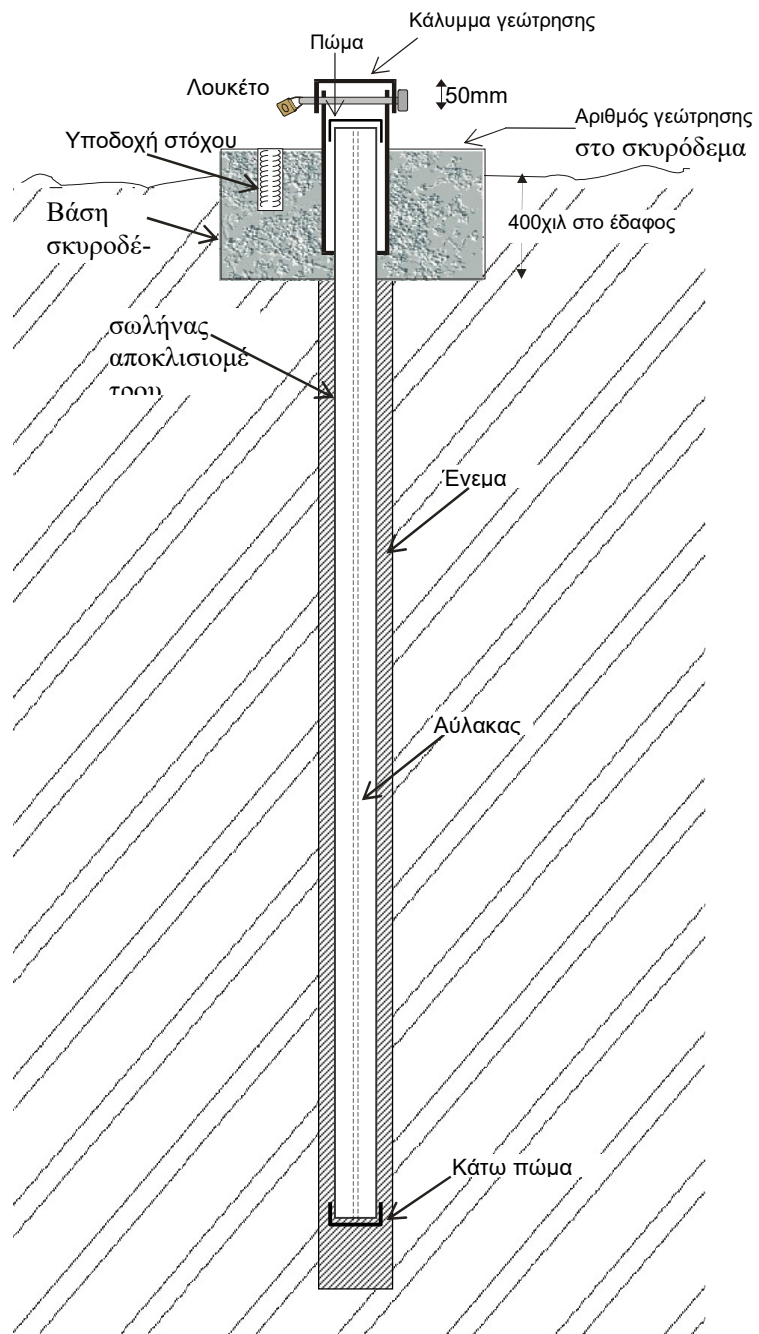
Σχήμα 3: Τυπική τομή αποκλισιομέτρου
